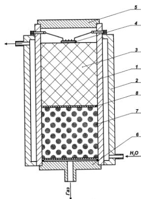
Рис. 1. СВС-реактор фильтрационного типа
